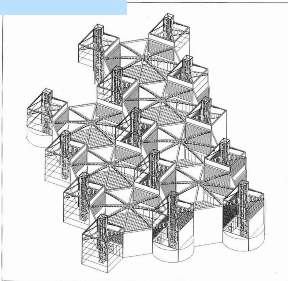
"näyttelypaviljonkien" rakennejärjestelmä (CAD-piirroksia)
