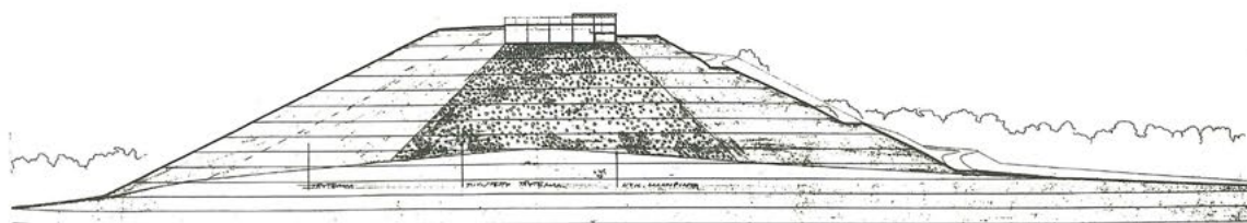
Maastoleikkaus 1:2500
