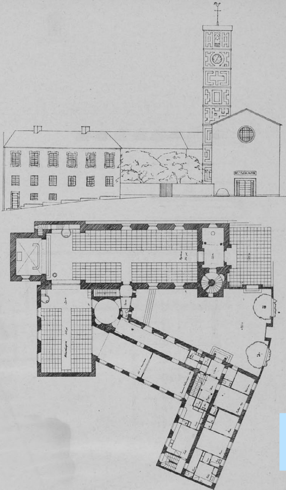
Kuva 60. Olaus Petrin kirkko, voittaneen kilpailuehdotuksen julkisivu ja pohjapiirros. Arkkitehti 12/1926, 201.
