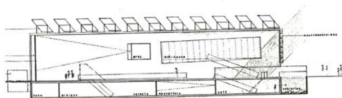
Leikkaus 1/750
