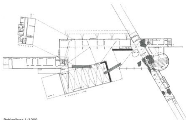
Pohjapiirros 1/1000
