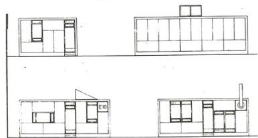
pohjat, julkisivut 1:300
