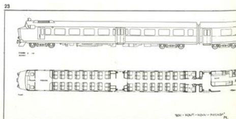
22–23. Pohja, julkisivuja ja leikkauksia / plans, elevations and sections 1/250
