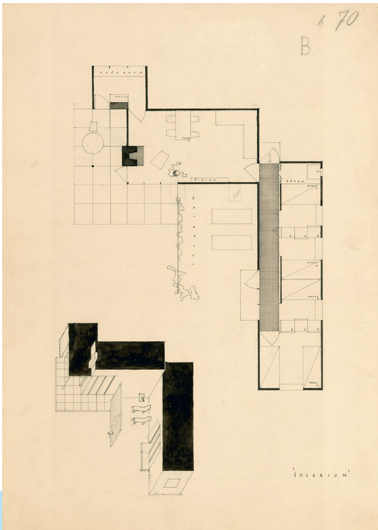
Kuva 43. Enso-Gutzeitin viikonloppumaja, kilpailuehdotuksen pohja- ja aksonometrinen piirros. Erik Bryggman, 1932.
